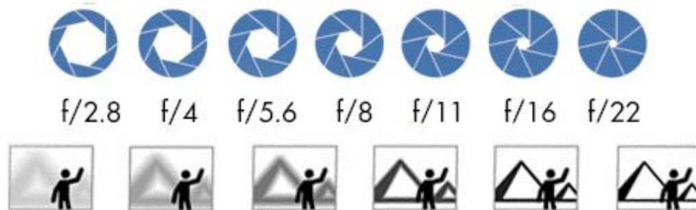
Blende und Schärfentiefe
